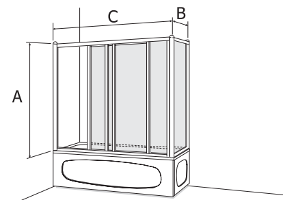
Posuvné dveře pro vyplnění niky nad vanou + pevná boční stěna + profil A505882
